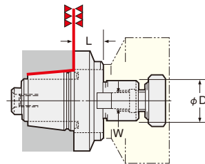
クイック型フェースミルアーバ(2面拘束型)
